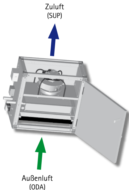
Abbildung zeigt das Gerät mit Anschlussseite rechts in Zulufttrichtung (Anschlussseite links in Zulufttrichtung ist spiegelbildlich)
