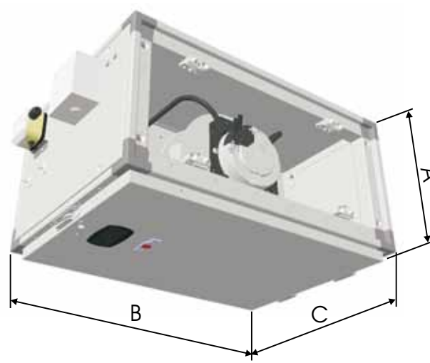
Abbildung zeigt das Gerät mit Anschlussseite rechts in Fortlufrichtung (Anschlussseite links in Fortlufrichtung ist spiegelbildlich)
