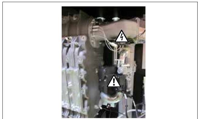
Bild: Zündtrafo, Hochspannungs-Zündelectrode, Gaskombiventil, Gasdruckwächter, Ventilator, Brennkammer Gefahr durch elektrische Spannung, Gefahr von Vergiftung und Explosion durch ausströmendes Gas, Gefahr von Verbrennung durch heiße Bauteile.
