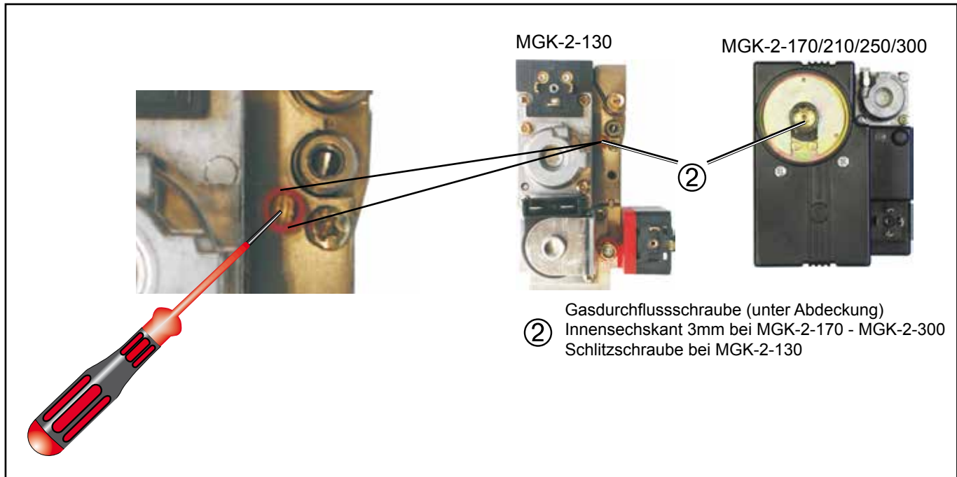
Bild: Gaskombiventil
