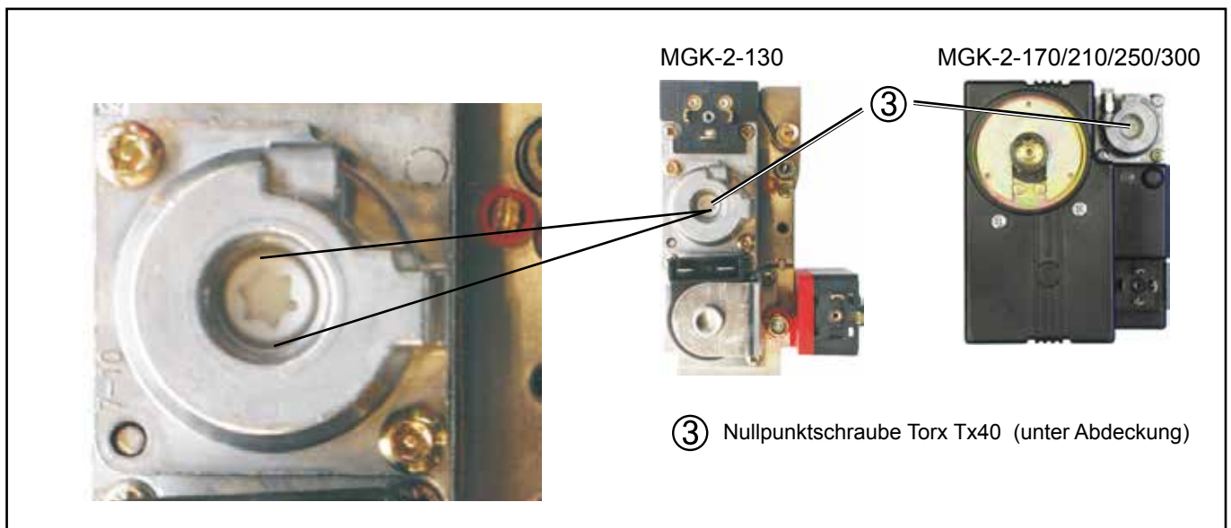
Bild: Gaskombiventil
