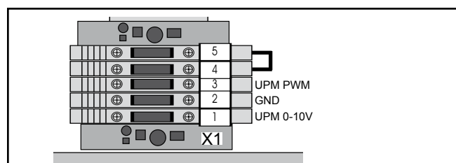
Bild: Anschluss Ausgang LP
